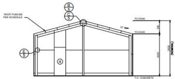
4 2 ENDWALL INTERIOR ELEVATION SCALE: 1 = 100
