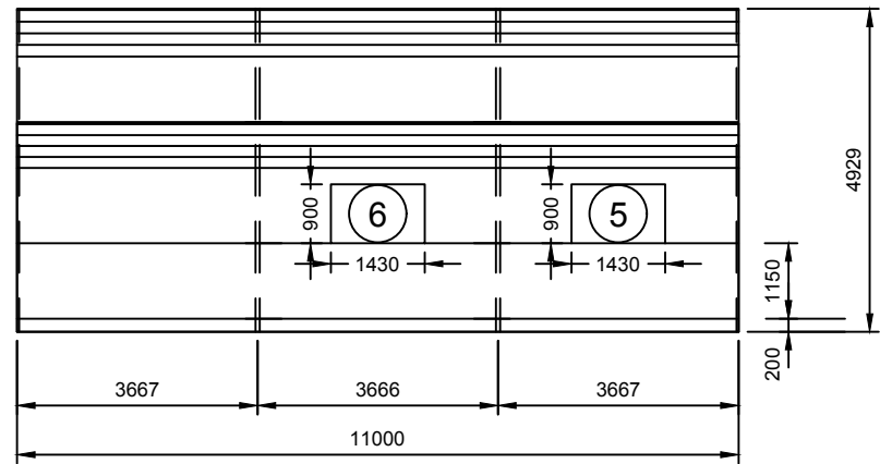
2 LEFT ELEVATION 3 SCALE: 1:125
