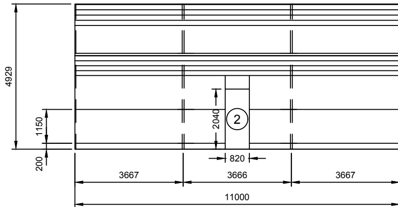
1 RIGHT ELEVATION 3 SCALE: 1:125
