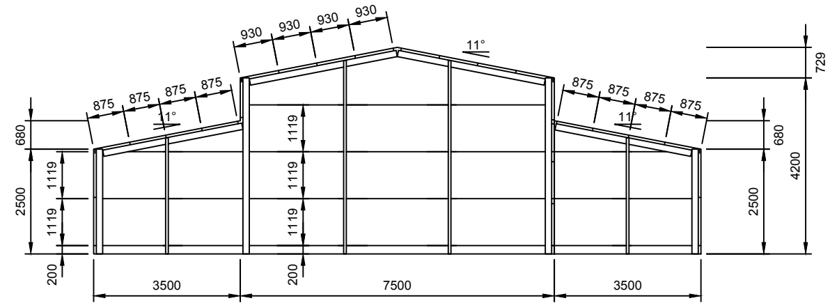
3 REAR ELEVATION 3 SCALE: 1:125
